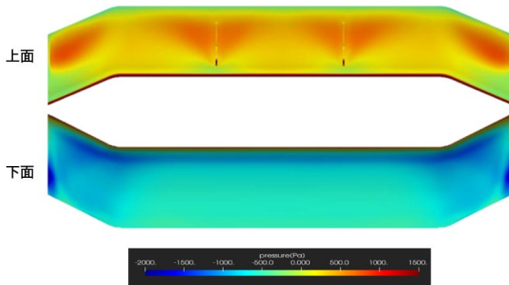
ウイング本体の圧力分布 (迎角 11度、車速 160km/h)
